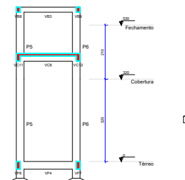
CORTE B-B Escala 1:50
