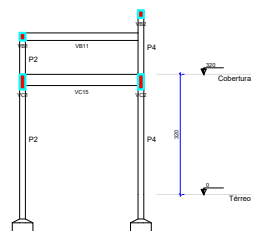
CORTE D-D Escala 1:50
