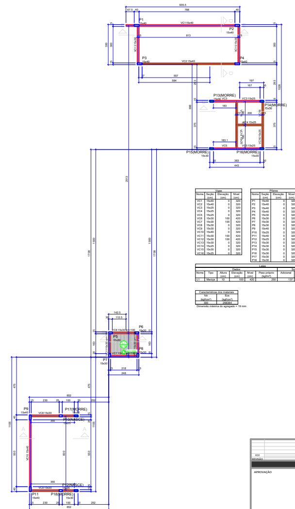
FORMA DO PAVIMENTO COBERTURA (NÍVEL 320) Escala 1:20
