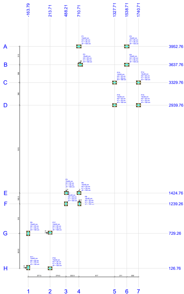
PLANTA DE LOCAÇÃO Escala 1:100
