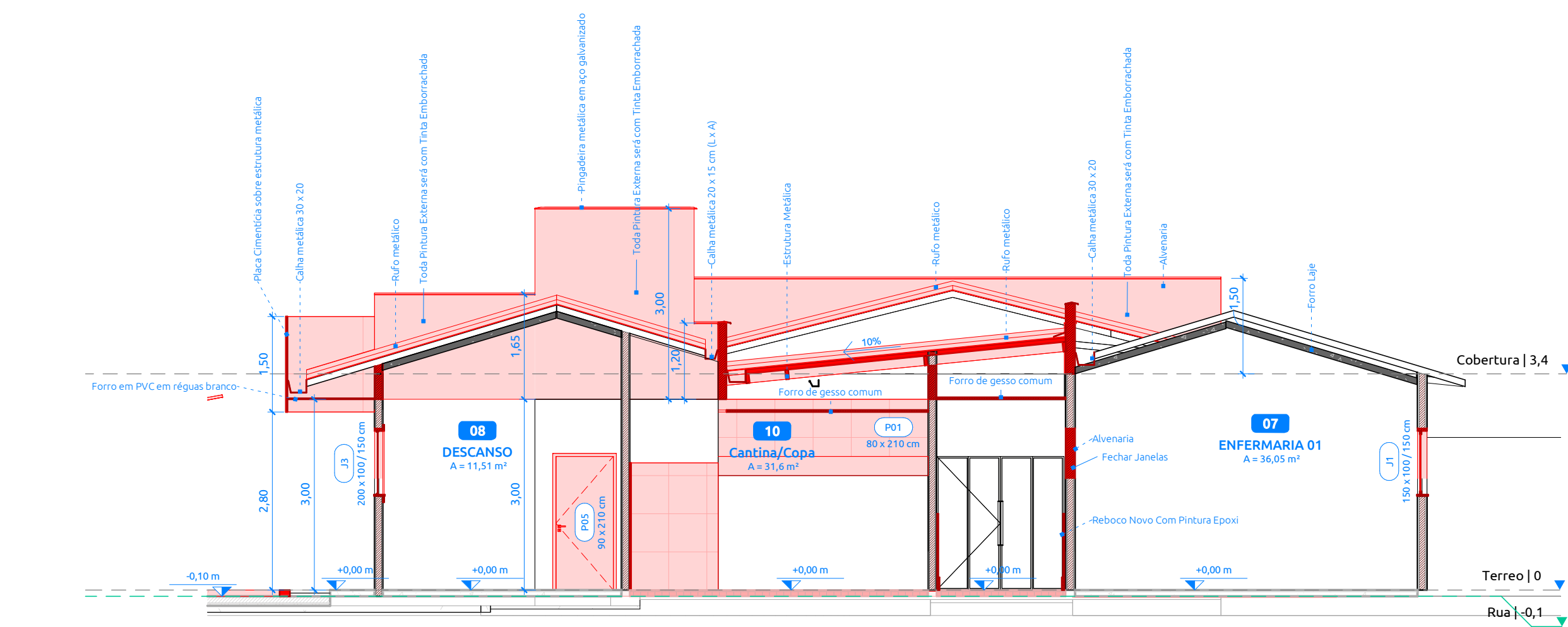
1 CORTE A CONSTRUÇÃO ESCALA: 1:75
