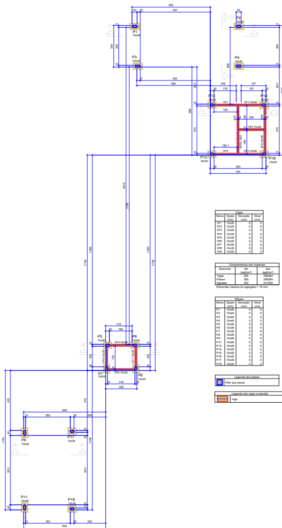
FORMA DO PAVIMENTO TÉRREO (NÍVEL 0) Escala 1:20
