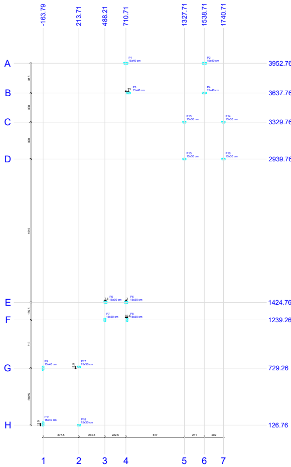
PLANTA DE CARGAS Escala 1:100
