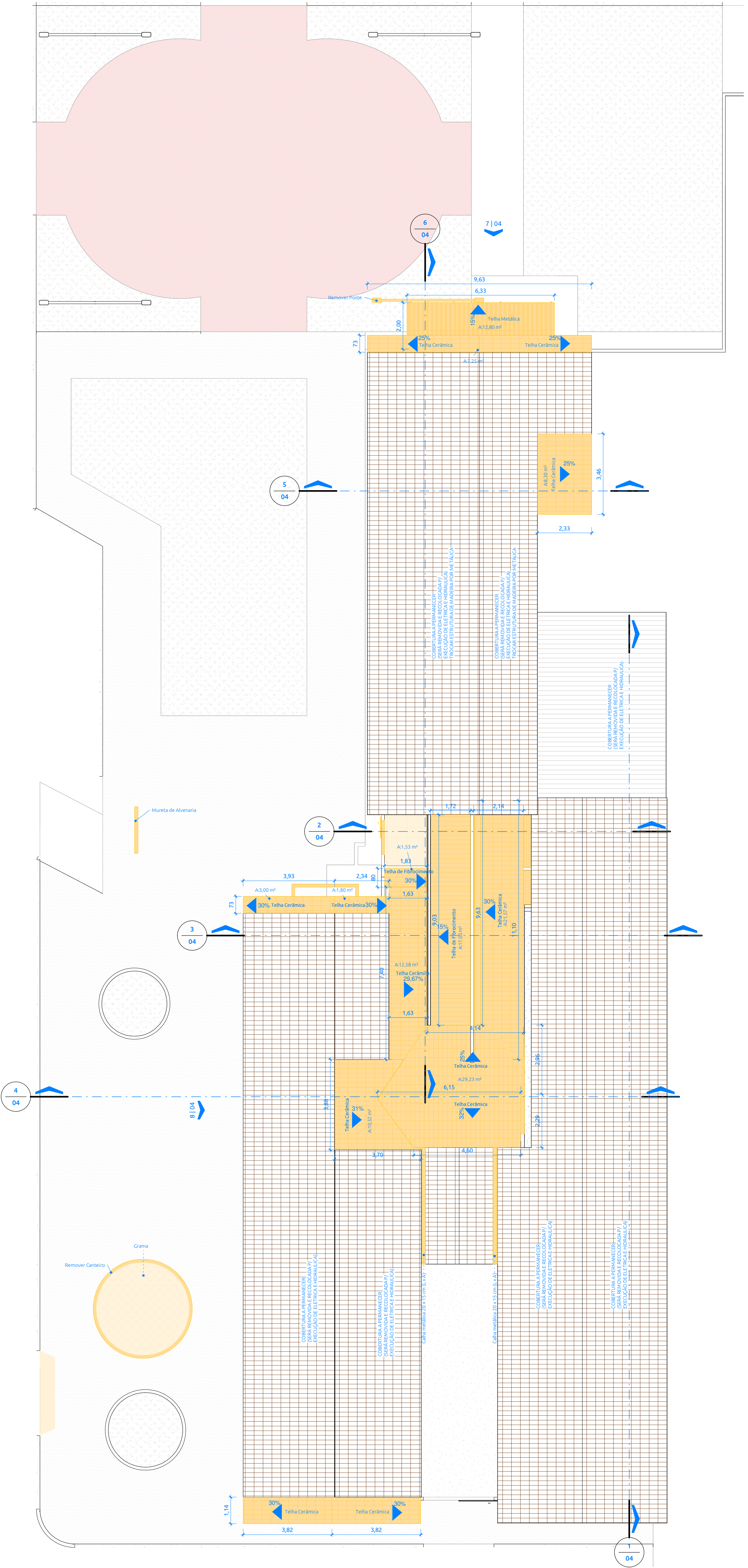
2 Cobertura Demolição ESCALA: 1: 100
